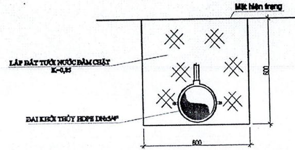
MẶT CẮT MƯỜNG BẮT ĐẠI KHỞI THỦY (KHÔNG TỈ LỆ)
