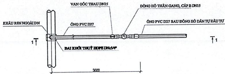
MẶT BẰNG CHI TIẾT LẮP ĐỒNG HỒ NƯỚC HỘ DẪN DN15 (KHÔNG TỈ LỆ)
