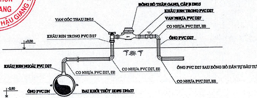
MẶT CẮT 1-1
